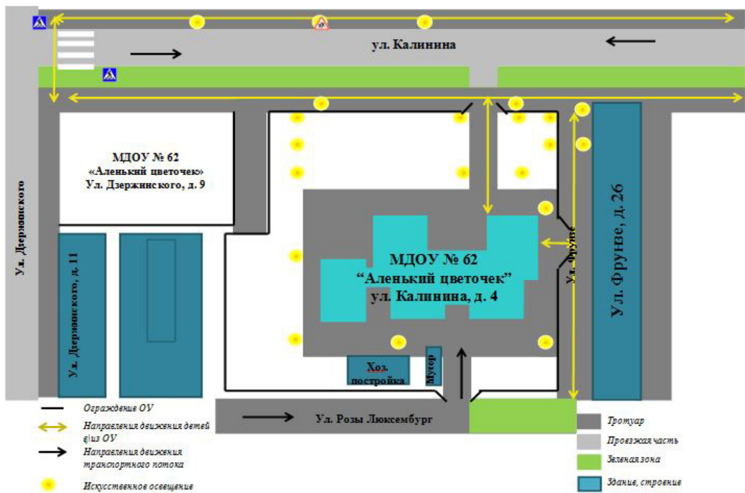
Схема организации дорожного движения со знаками и освещением.
