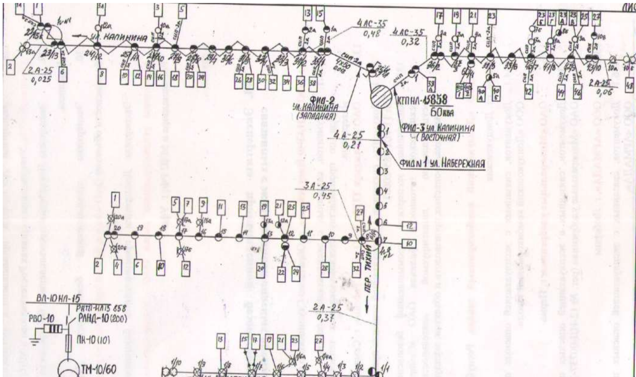
Обосновывающие материалы. Схема электроснабжения (лист № 37) ст. Новолешковская. Масштаб 1:5000
