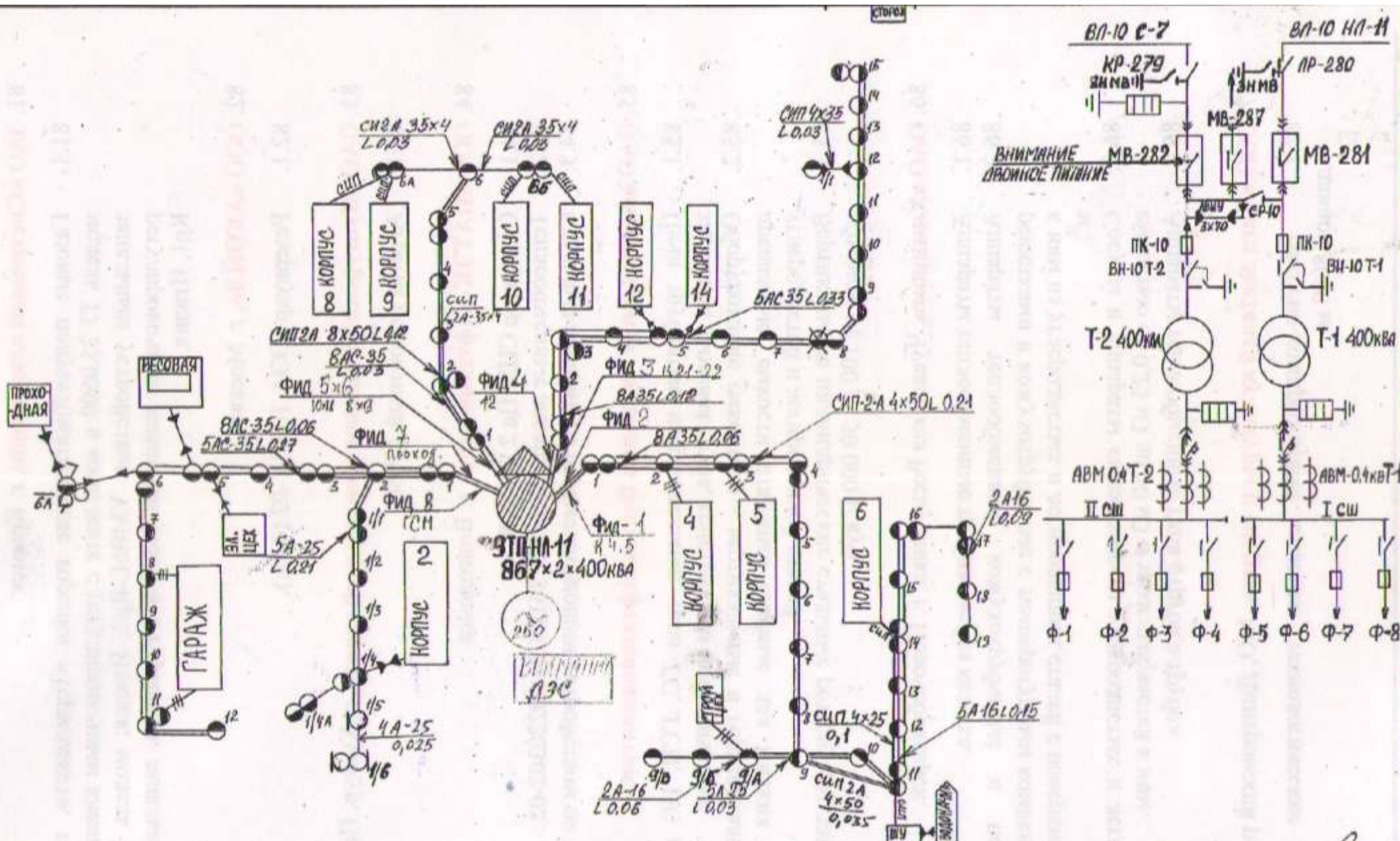
Обосновывающие материалы. Схема электроснабжения (лист № 43) ст. Новолешковская. Масштаб 1:5000
