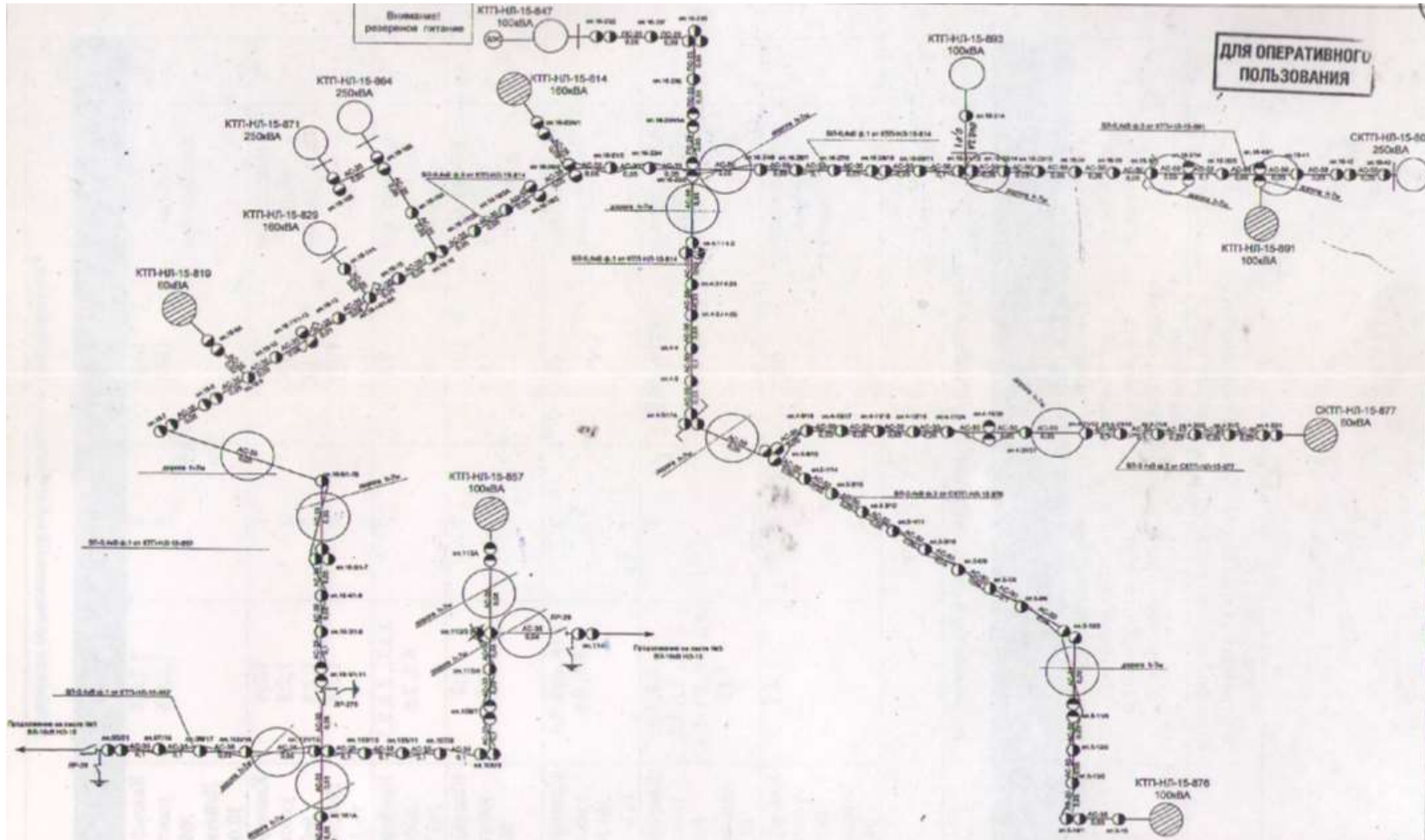
Обосновывающие материалы. Схема электроснабжения (лист № 61) ст. Новолешковская. Масштаб 1:5000
